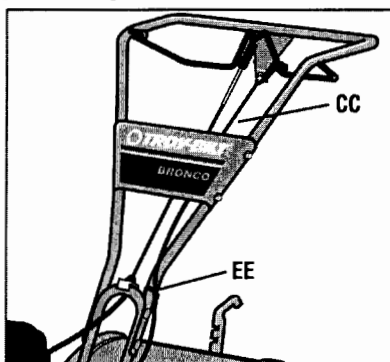
Illustration 2-9 : Disposer le câble d'embrayage de marche arrière (CC) tel qu'illustré. Fixez à l'aide d'une attache de câble (EE).
