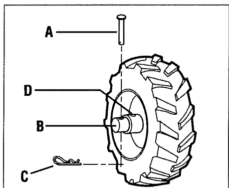
Illustration 3-3: Réglage ROUE LIBRE
