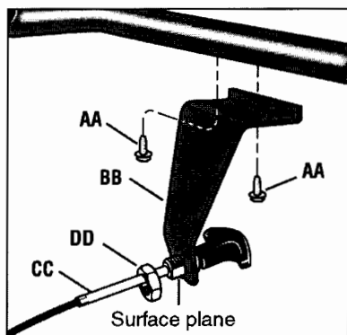
Illustration 2-8 : Installation du support de câble et du câble d'embrayage de marche arrière
