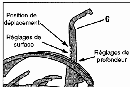
Illustration 3-5 : Levier du dispositif de terrage (G)
