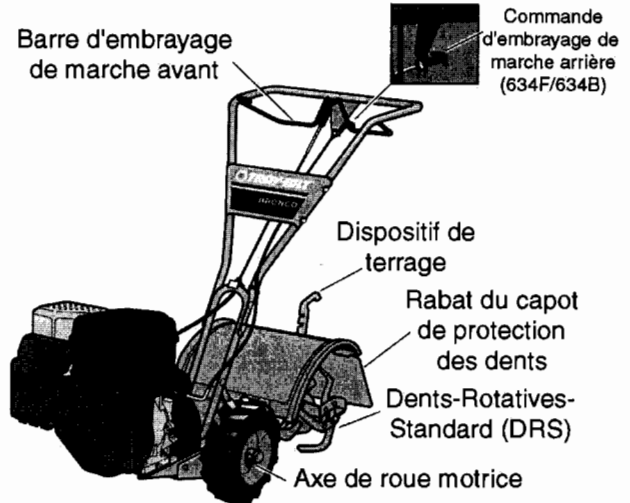
Illustration 1-1 : Commandes et fonctions du motoculteur (modèle illustré 5,5 Hp). Se reporter au manuel de l'utilisateur du moteur pour la description des commandes du moteur.
