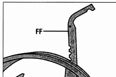
Illustration 2-10 : Réglage du levier du dispositif de terrage
