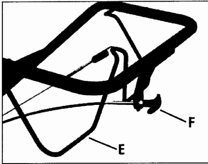
Illustration 3-4 : Tous les modèles sont munis d'une barre d'embrayage de marche avant (E). Seul les modèles 634A sont munis de la commande d'embrayage de marche arrière (F).
