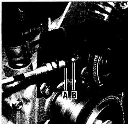
Illustration 5-5 : Mesurer la longueur du fil métallique pour vérifier la tension de la courroie de marche arrière
