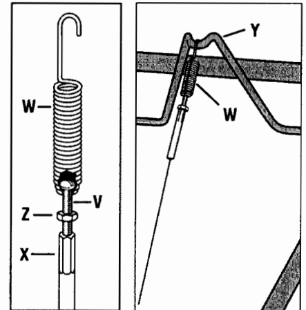
Illustration 2-5 : Ressort de câble et tendeur
