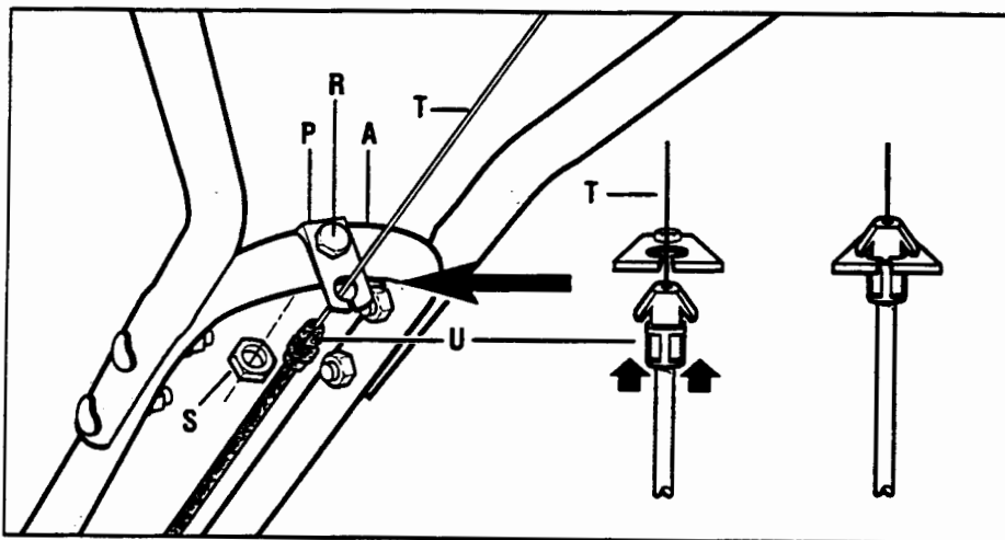
Illustration 2-4 : Installation du support de câble et du câble d'embrayage avant
