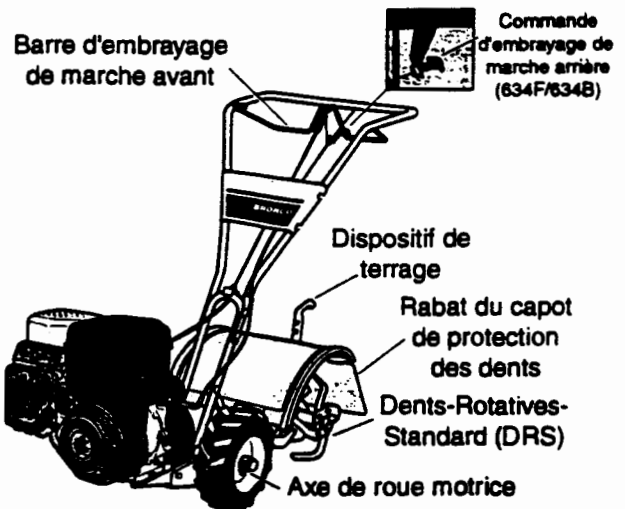
Illustration 1-1: Commandes et fonctions du motoculteur (modèle illustré 5,5 Hp). Se reporter au manuel de l'utilisateur du moteur pour la description des commandes du moteur.
