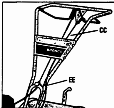
Illustration 2-9 : Disposer le câble d'embrayage de marche arrière (CC) tel qu'illustré. Fixer à l'aide d'une attache de câble (EE).
