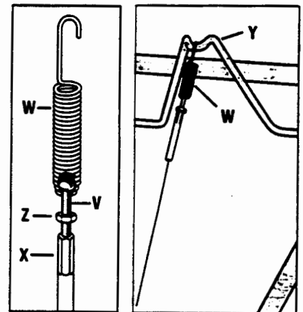
Illustration 2-5 : Ressort de câble et tendeur
