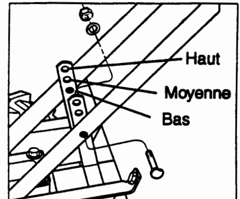
Illustration 3-6 : Réglage de la hauteur du guidon
