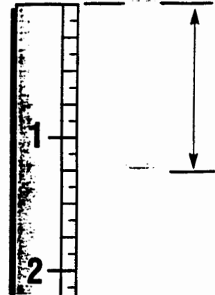
Illustration 2-1 : Pour déterminer la longueur des vis, placer la vis sur le gabarit, telle qu'illustrée, et mesurer la distance entre le bas de la vis et la tête de la vis.
