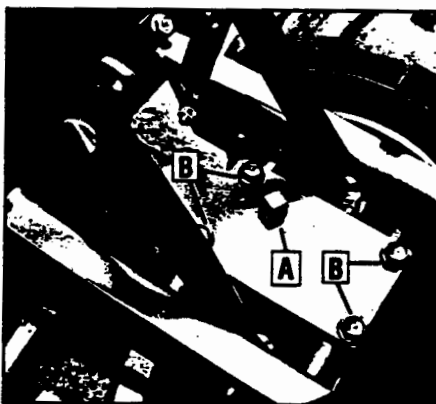
Illustration 5-2 : Retirer le bouchon de remplissage (A) pour vérifier le niveau d'huile et pour ajouter de l'huile pour transmission. Retirer les quatre vis du protecteur (B) pour vidanger l'huile.
